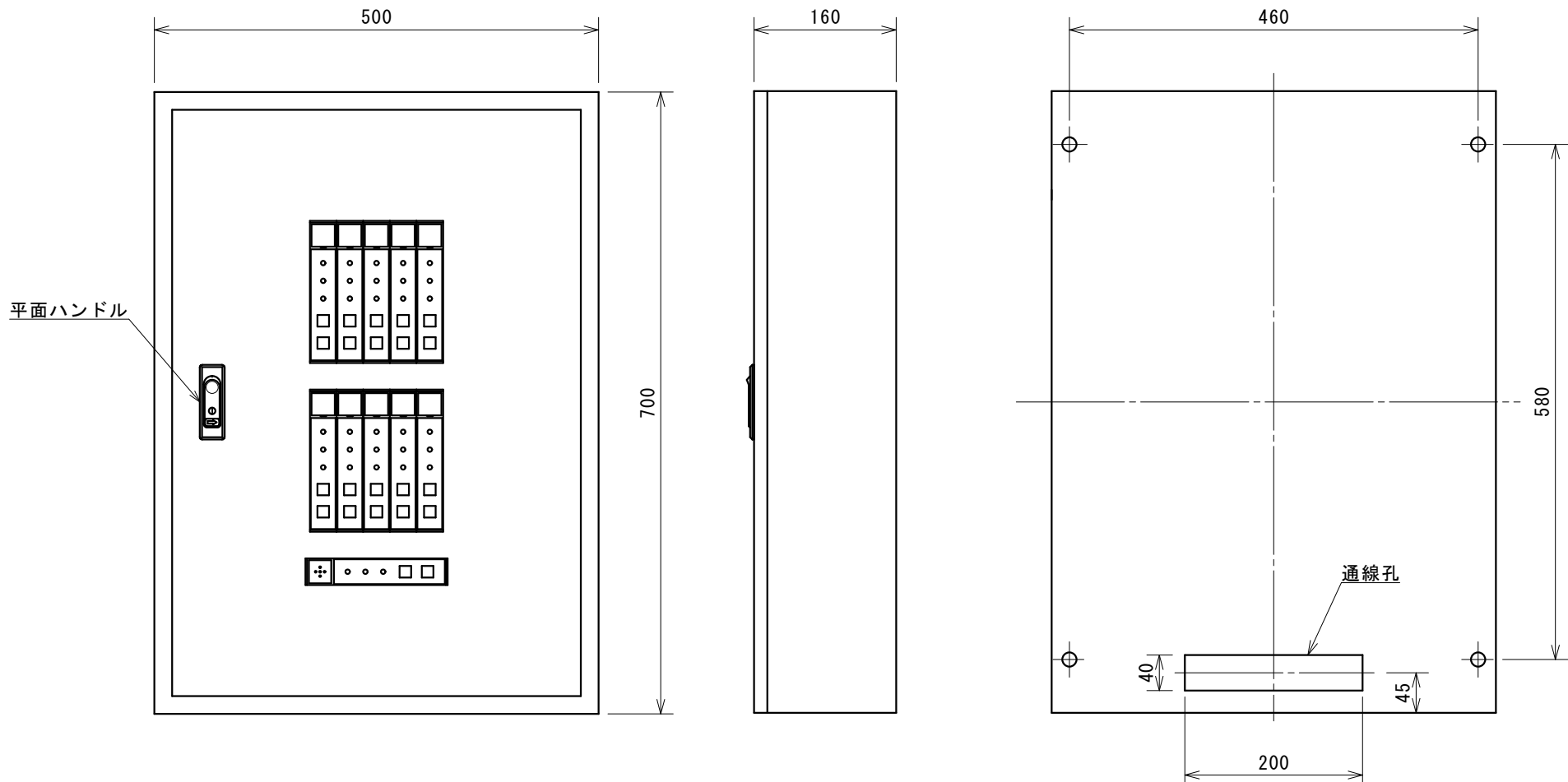
選択パネル詳細（１：３）
