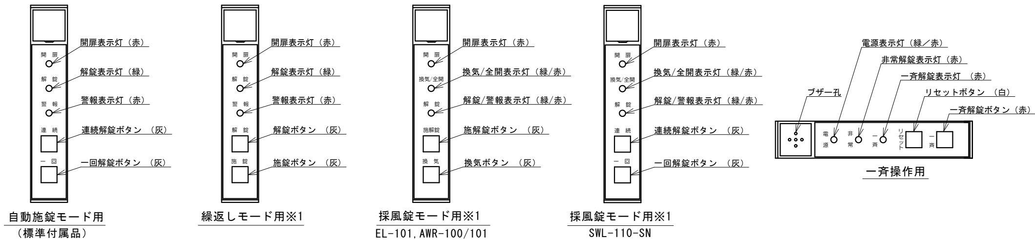
選択パネル詳細（１：３）
