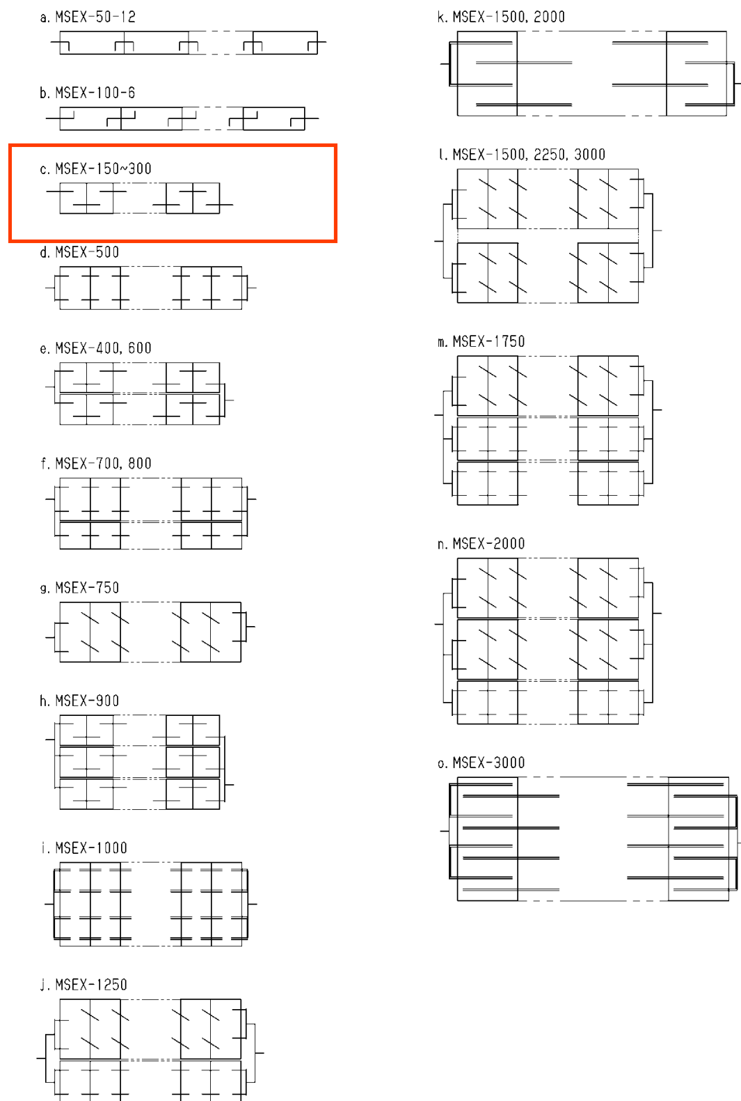
図2 蓄電池接続略図
