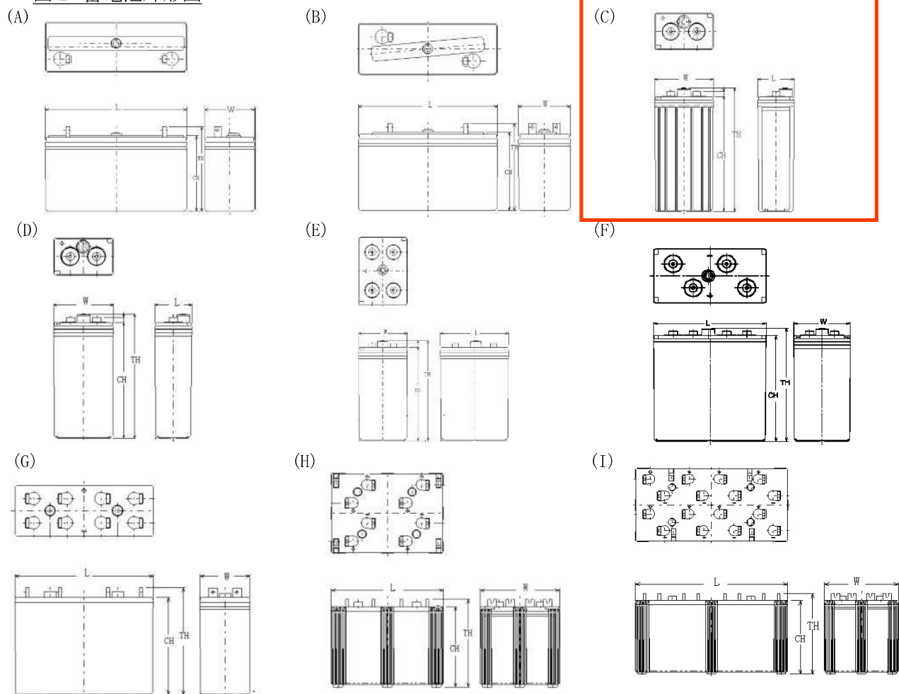
図1 蓄電池外形図
