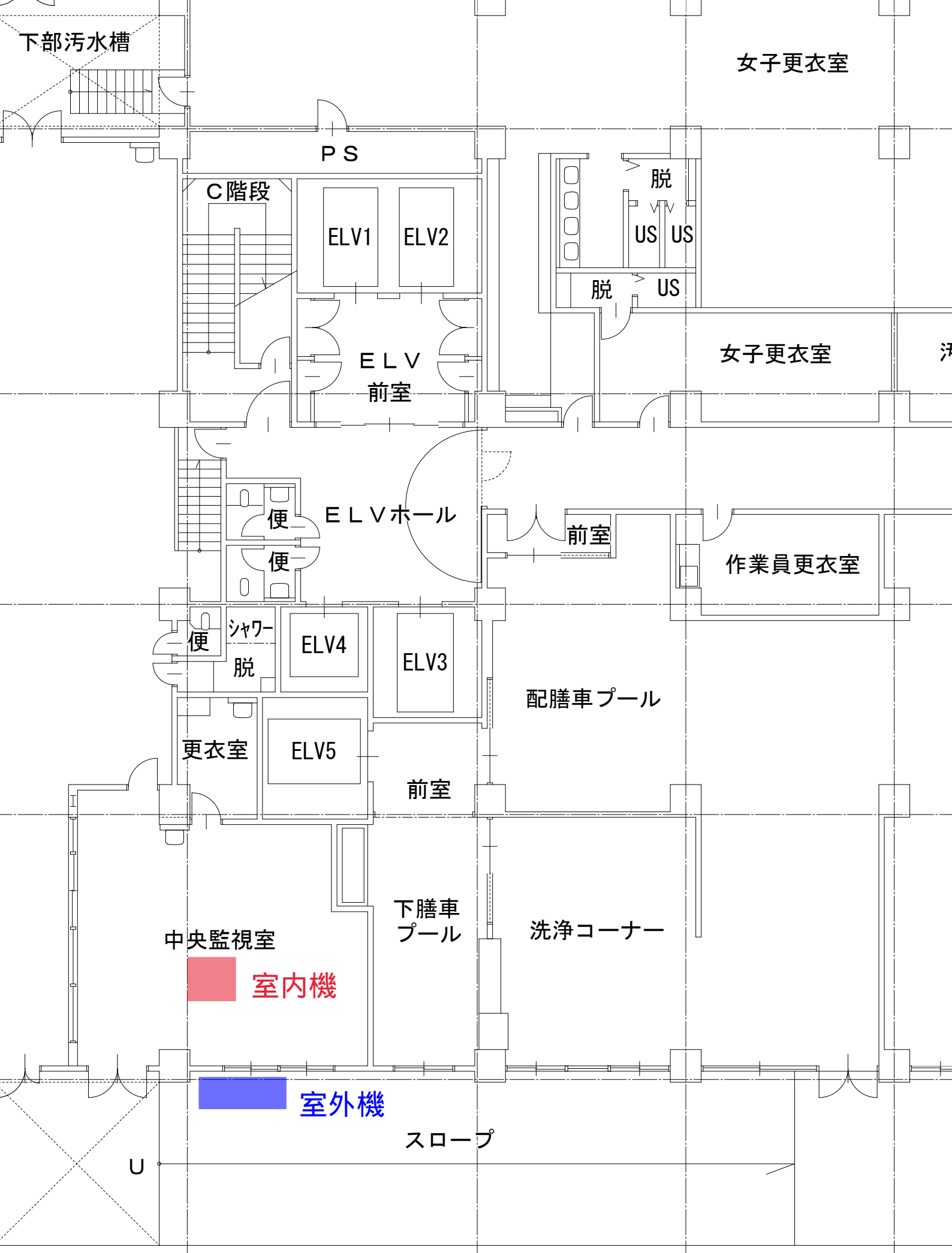
地階平面図
