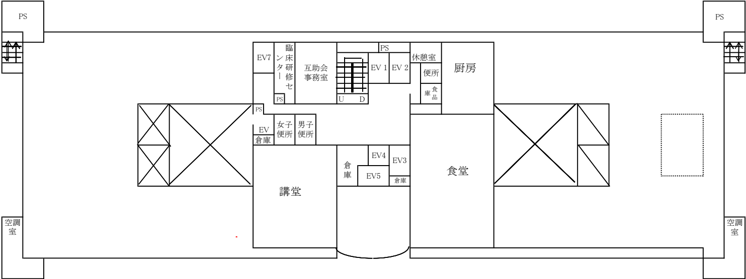
7F配置図
